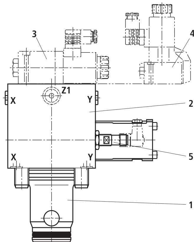
Beispiel: Typ LFA 40 EWMA-7X/..Q6G24..
