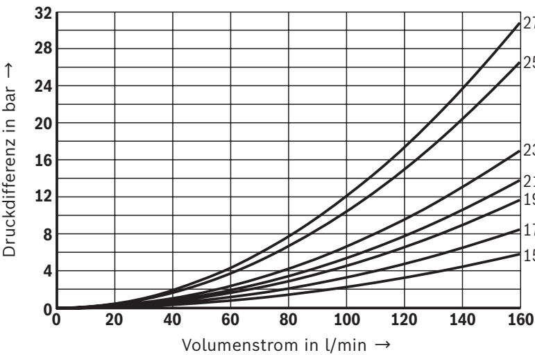
\Delta p - q_v -Kennlinien
